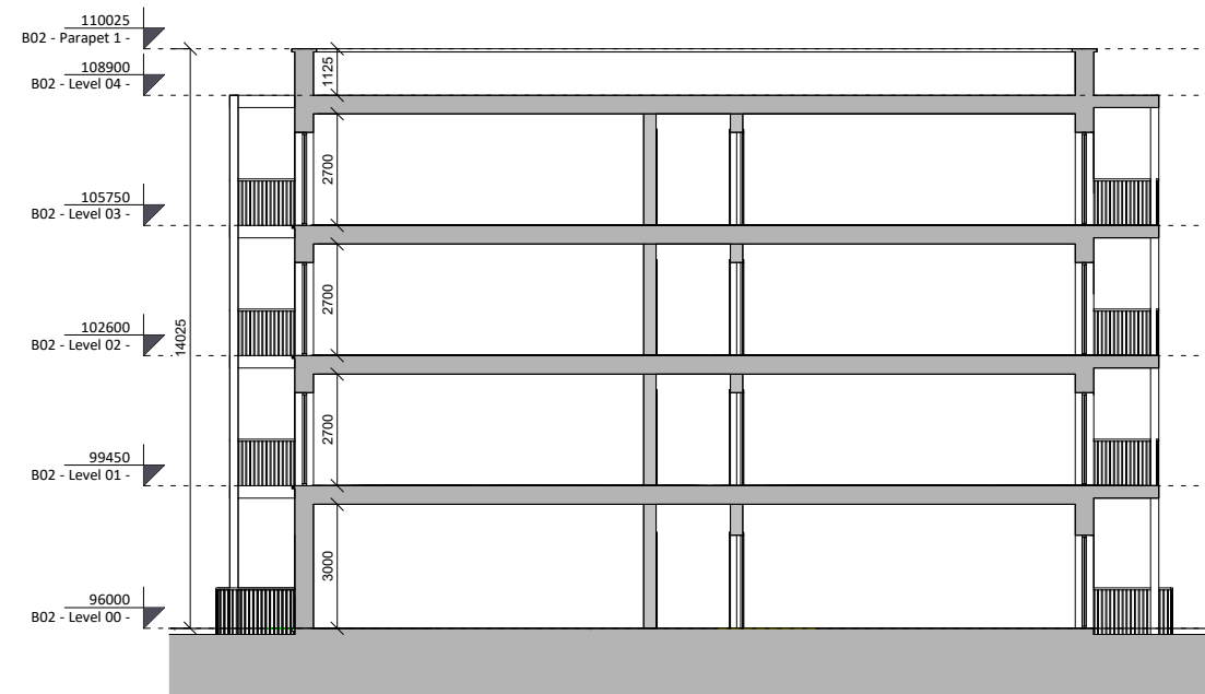
③ Block 02 - Section A-A 1 : 200
